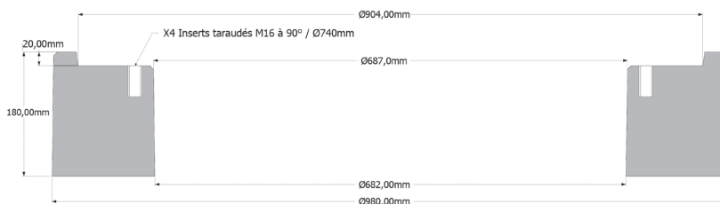
Coupe dalle de répartition Ø980
