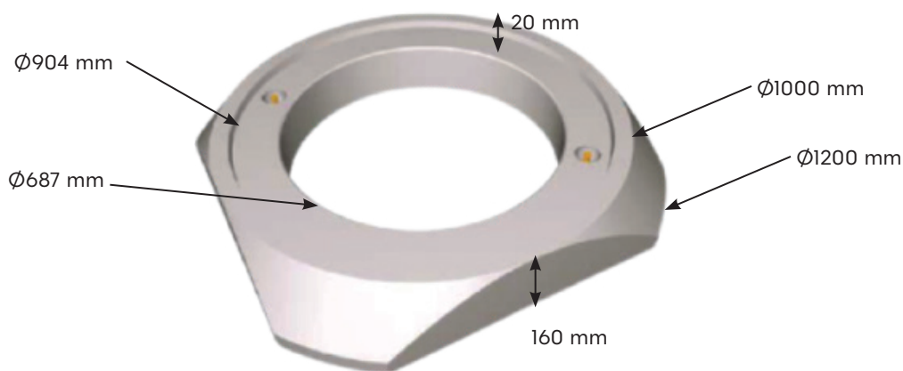
Dalle de répartition CIRCLE MAXI Réf. DALCIRCLEMAXI
